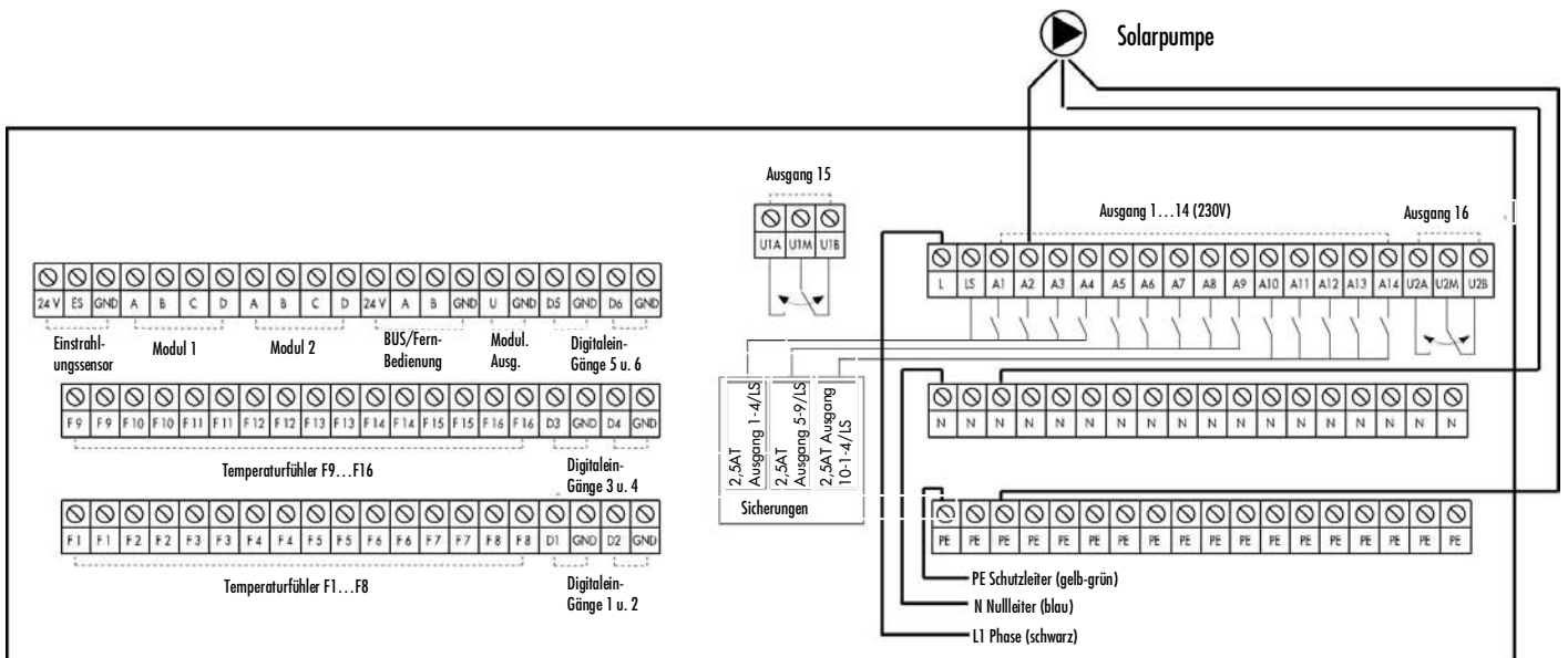
Abbildung 2: Anschlussplatine des CONTROL 701 mit Anschlussbeispiel für Solarpumpe
