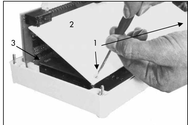
Abbildung 4: Montage der PC- Schnittstelle
