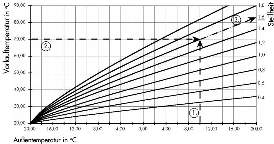
Heizkennlinien
