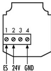
Abbildung 3: Klemmenbelegung des Einstrahlungssensors ES3
