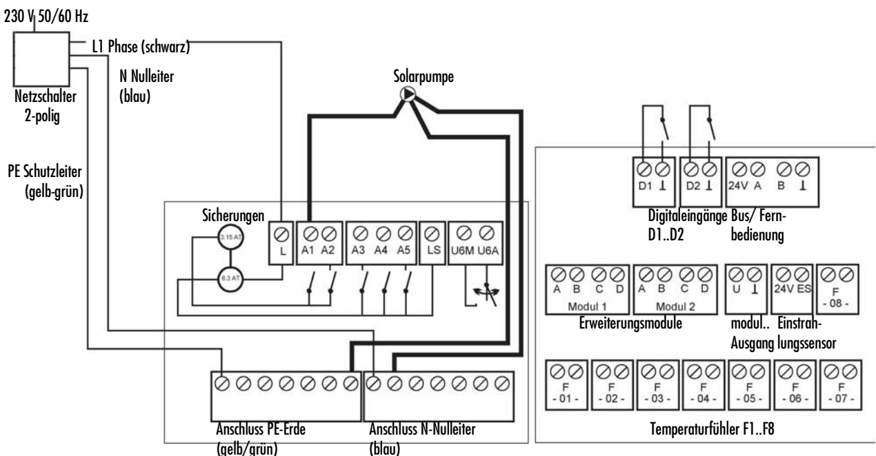
Abbildung 2: Anschlussplatine des CONTROL 601 mit Anschlussbeispiel für Solarpumpe
