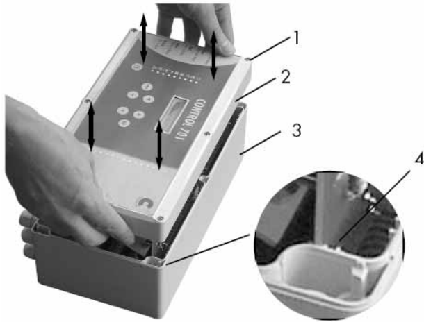
Abbildung 1: Gehäuse CONTROL 701
