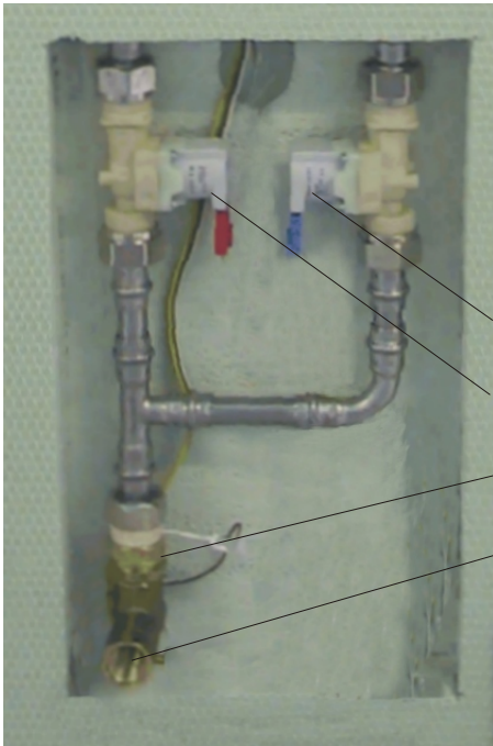
Sifon, Abfluss
