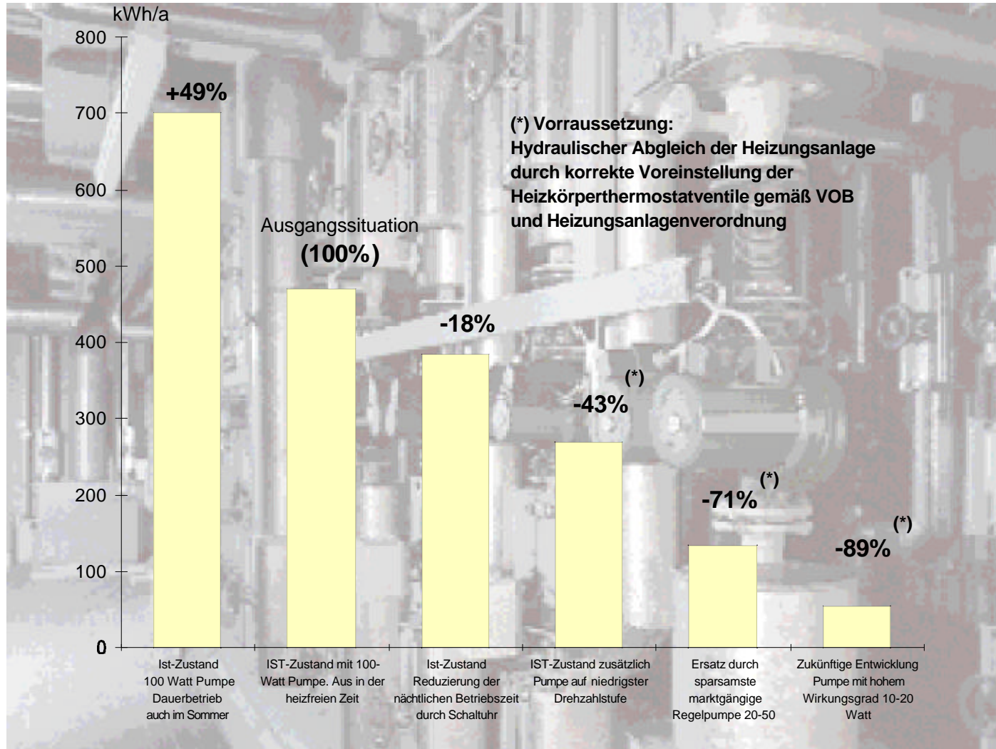
Stromverbrauch der Heizungsumwälzpumpe für ein Einfamilienhaus
