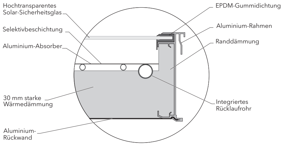
Abb. 2 Kollektoraufbau
