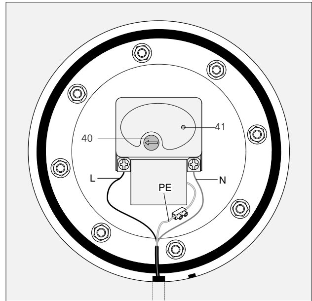
Abb. 13 Elektrische Anschlüsse am Elektroheizstab bei entferntem Speicherdeckel: L Außenleiter („Phase“); N Neutraleiter; PE Schutzkontakt; 40 Drehregler zum Einstellen der Solltemperatur; 41 Reset-taste
