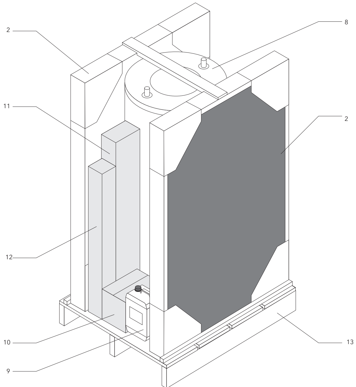
Abb. 9 Auslieferungszustand SECUterm 8 Speichereinheit; 2 Kollektoren (Beispiel SECUterm 300 P); 9 Behälter mit Solarkonzentrat; 10 Zubehörkarton; 11 und 12 Kartons Montagesystem (nur bei SECUterm 300 P); 13 Palette
