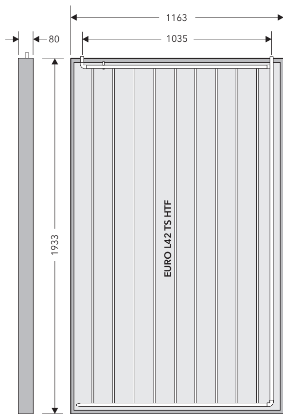
Abb. 3 Kollektorabmessungen (mm)
