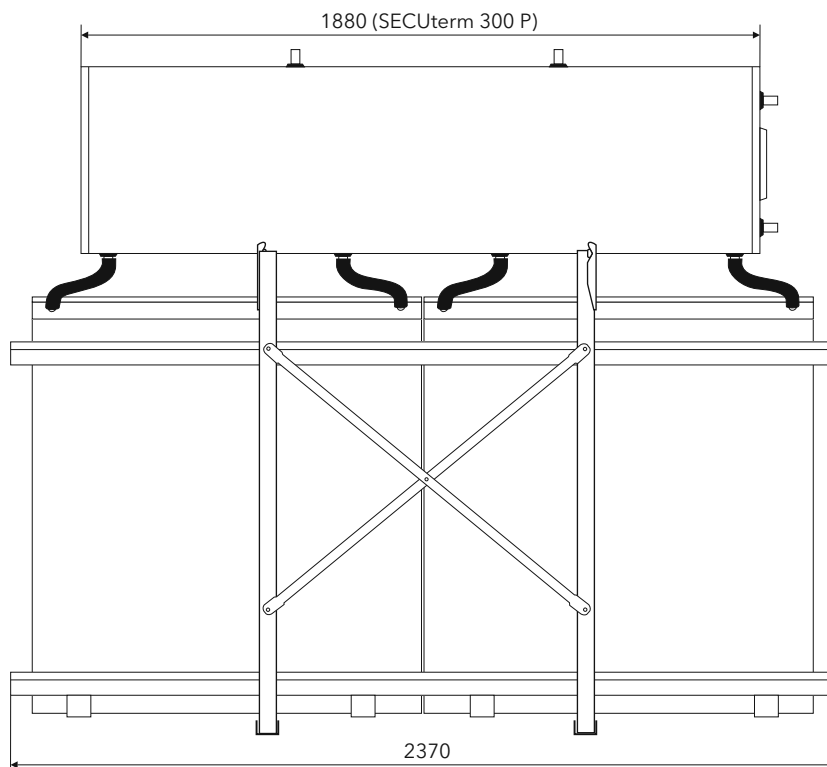
Abb. 4 Abmessungen SECUterm 160 P, 200 P und 300 P (mm)
