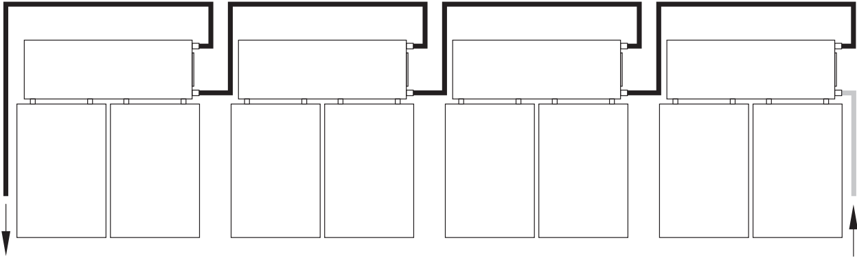
Abb. 7 Serielle Verschaltung von maximal 4 Anlagen; zu verwenden sind Rohrdurchmesser von 22 mm. Hinweis: Der Heizstab muss bei den ersten beiden Anlagen ausgeschaltet bleiben
